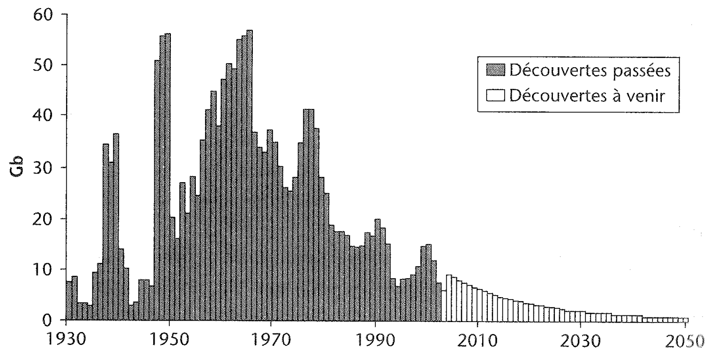
Figure 3.4 : Découvertes mondiales de pétrole (sources : ASPO et Exxon Mobil, 2002).
